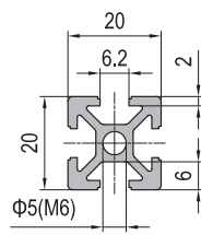
20x20 4 slots 20x20 4槽
