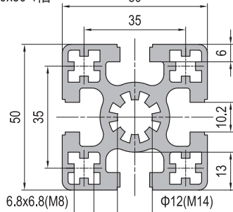
50x50 4 slots 50x50 4槽
