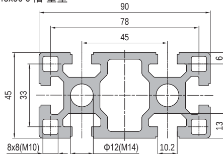
45x90 6 slots Heavy 45x90 6槽 重型
