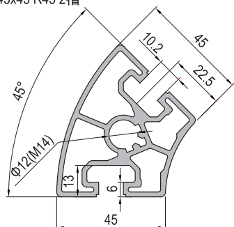
45x45 R45 2 slots 45x45 R45 2槽
