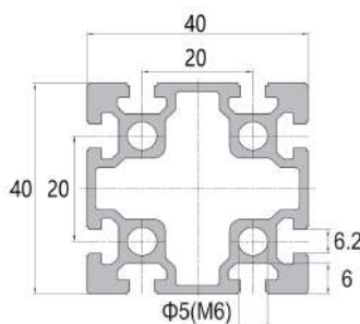
40x40 8 slots 40x40 8槽
