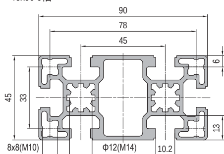
45x90 6 slots 45x90 6槽
