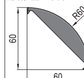
Bracket Cap-PG30-6060 角铝扣盖-30系列-6060
