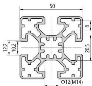
50x50 4 slots Light 50x50 4槽 轻型
