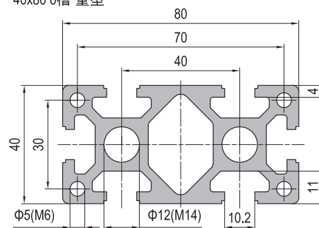
40x80 6 slots Heavy 40x80 6槽 重型
