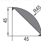
Bracket Cap-PG45-4545 角铝扣盖-45系列-4545
