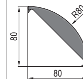
Bracket Cap-PG40-8080 角铝扣盖-40系列-8080
