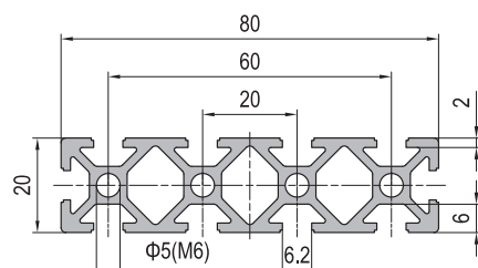
20x80 10 slots 20x80 10槽
