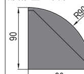
Bracket Cap-PG45-4590 角铝扣盖-45系列-4590
