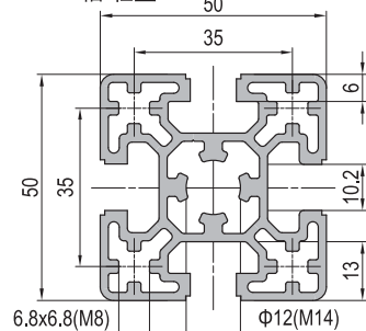
50x50 4 slots Light 50x50 4槽 轻型
