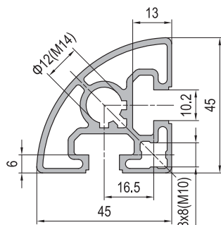
45x45 4 slots Super Light 45x45 4槽 超轻型
