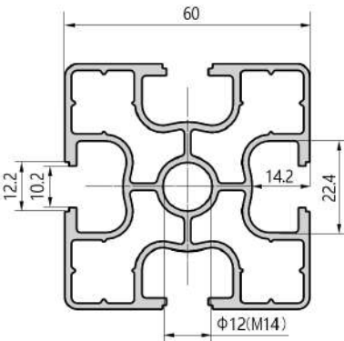
60x60 4 slots Super Light 60x60 4槽 超轻型
