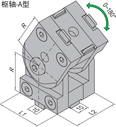
Joint-Type B 枢轴-B型
