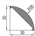
Bracket Cap-PG30-3030 角铝扣盖-30系列-3030
