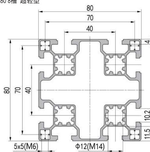
80x80 8 slots Super Light 80x80 8槽 超轻型
