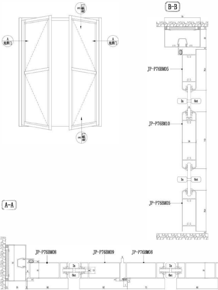
JP-YN70B Casement Door - Non Thermal Break
